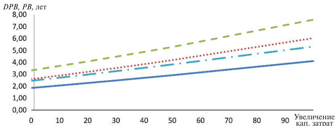
Рис. 5. Чувствительность проекта к увеличению капитальных затрат проектов: - · · · - DPB Q_{\text{ТНУ}} = 50 МВт; — — — PB Q_{\text{ТНУ}} = 50 МВт; · · · · · - DPB Q_{\text{ТНУ}} = 2 МВт; - - - - - PB Q_{\text{ТНУ}} = 2 МВт
